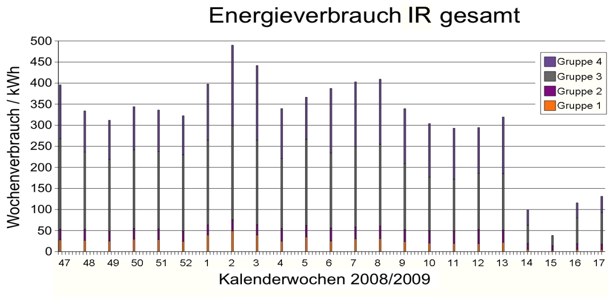
Bild 4.7: Wochen-Energieverbrauch der IR-Heizung
