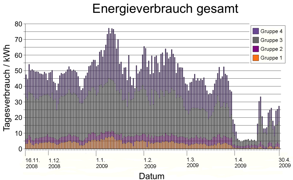
Bild 4.5: Gesamter Tages-Energieverbrauch aller Gruppen
