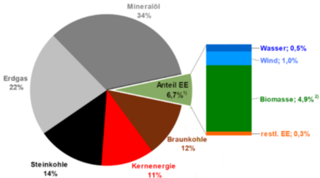
Bild 1.3: Primärenergieverbrauch Deutschland
