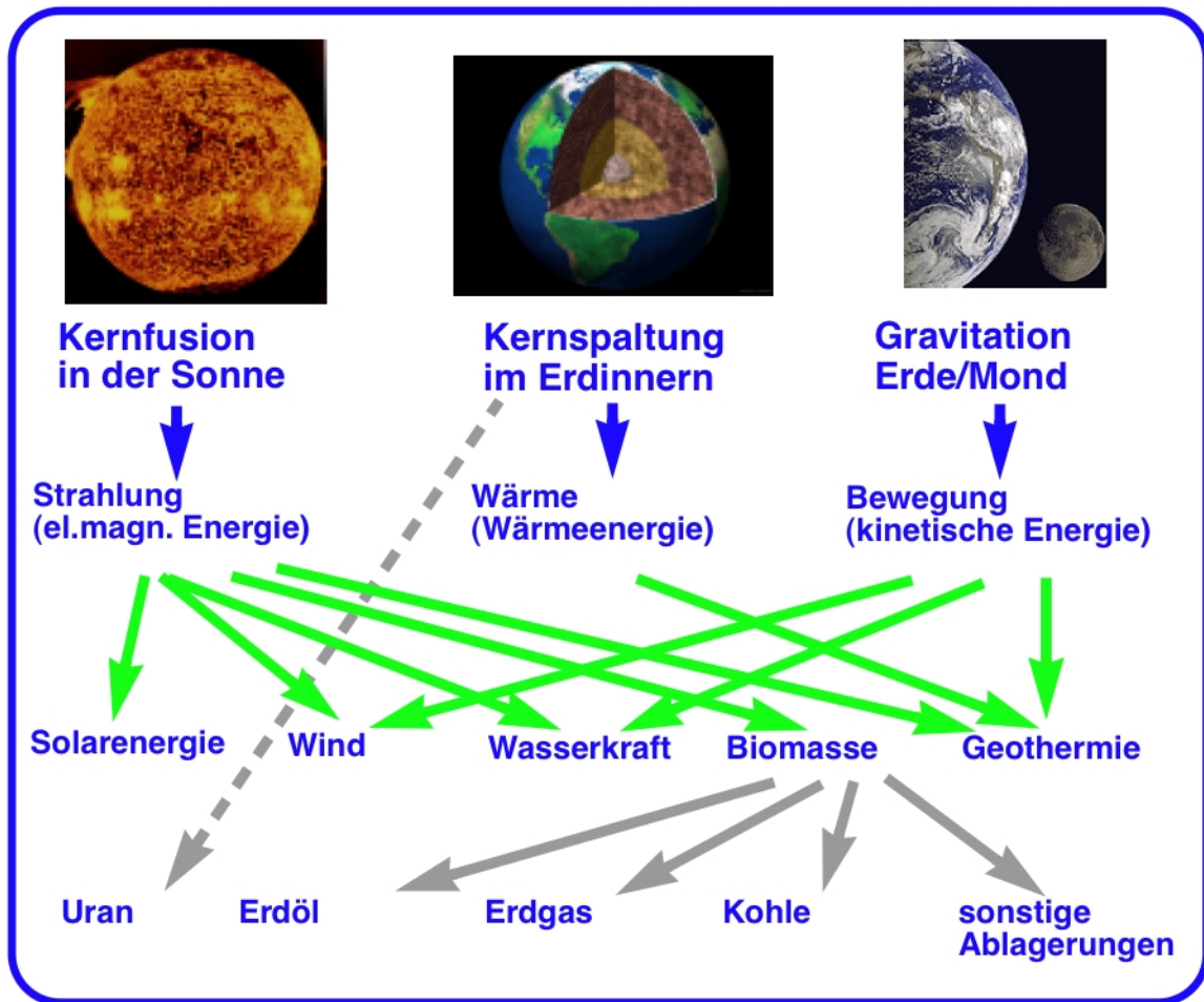
Bild 1.2: Nutzbares Energiespektrum
