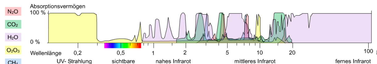
Bild 1.6: Absorptionsspektren verschiedener Stoffe in Luft
