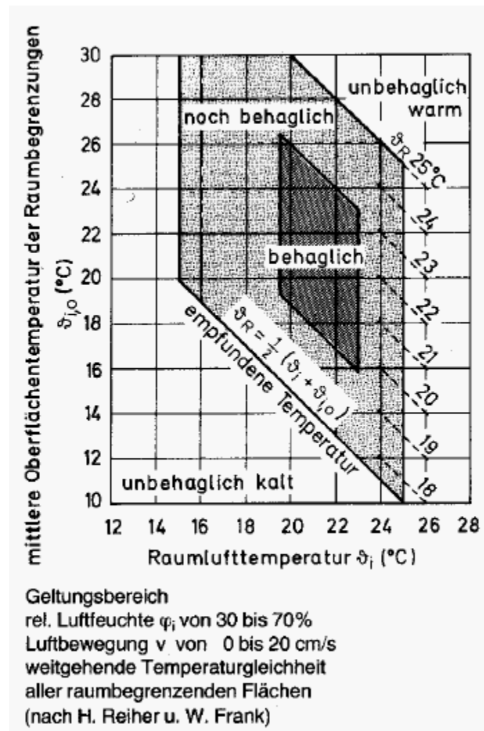
Bild 1.7: Strahlungstemperatur-Lufttemperatur-Diagramm
