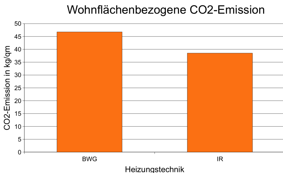
Bild 5.2: Vergleich der CO 2 -Emissionen
