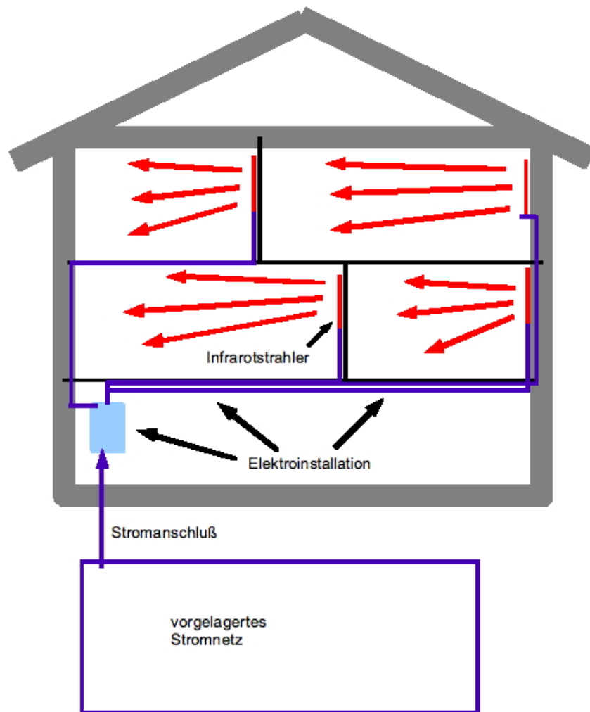
Bild 3.2: Prinzipieller Aufbau einer Infrarotheizung
